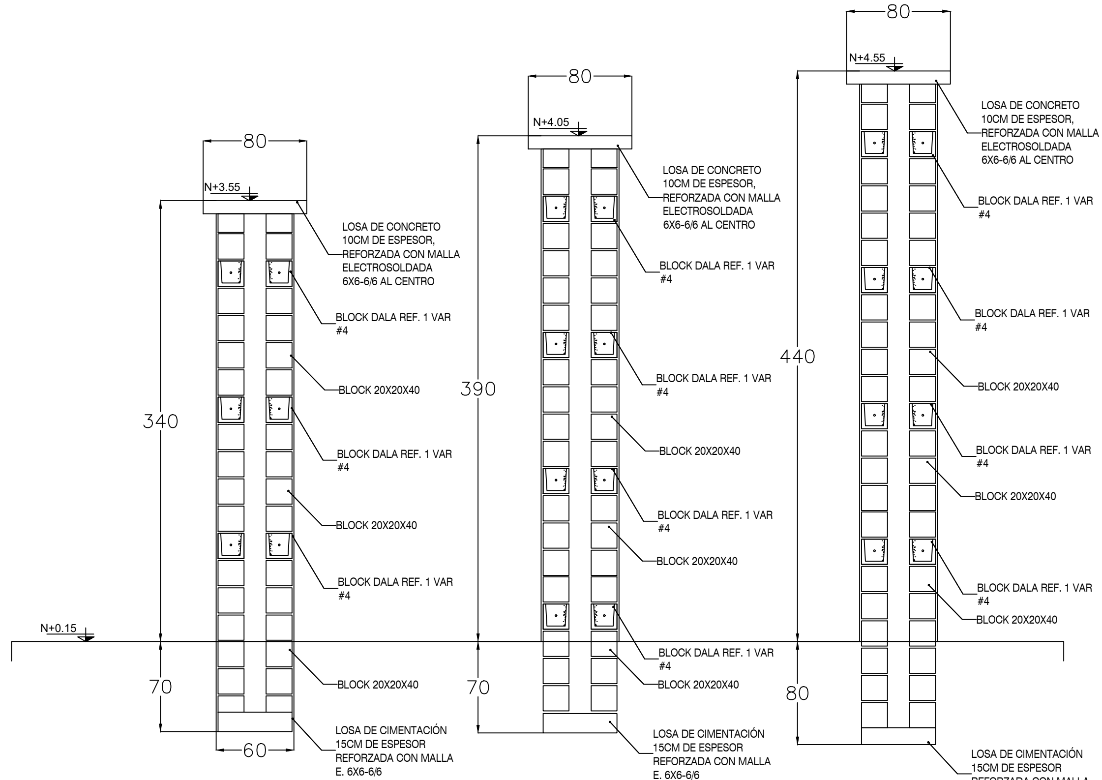
CORTE ESTRUCTURA DE PÓRTICO PR-01A, PR-01B Y PR-01C. ALZADO
