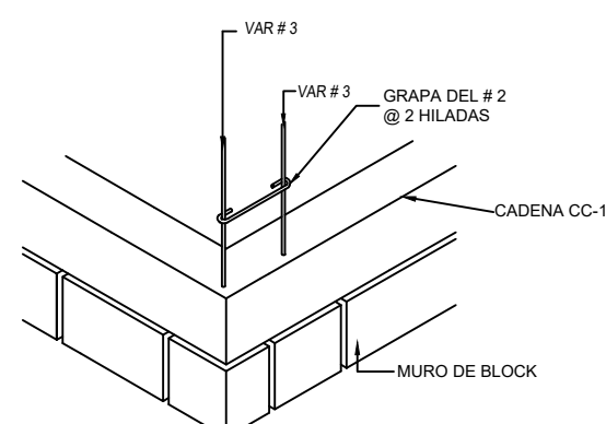
DETALLE DE ANCLAJE DE CASTILLO EN ESQUINA O INTERSECCIÓN ISOMETRICO-ESCALA 1:20
