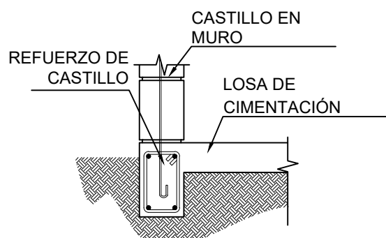
ANCLAJE DE REFUERZO DE MUROS ALZADO
