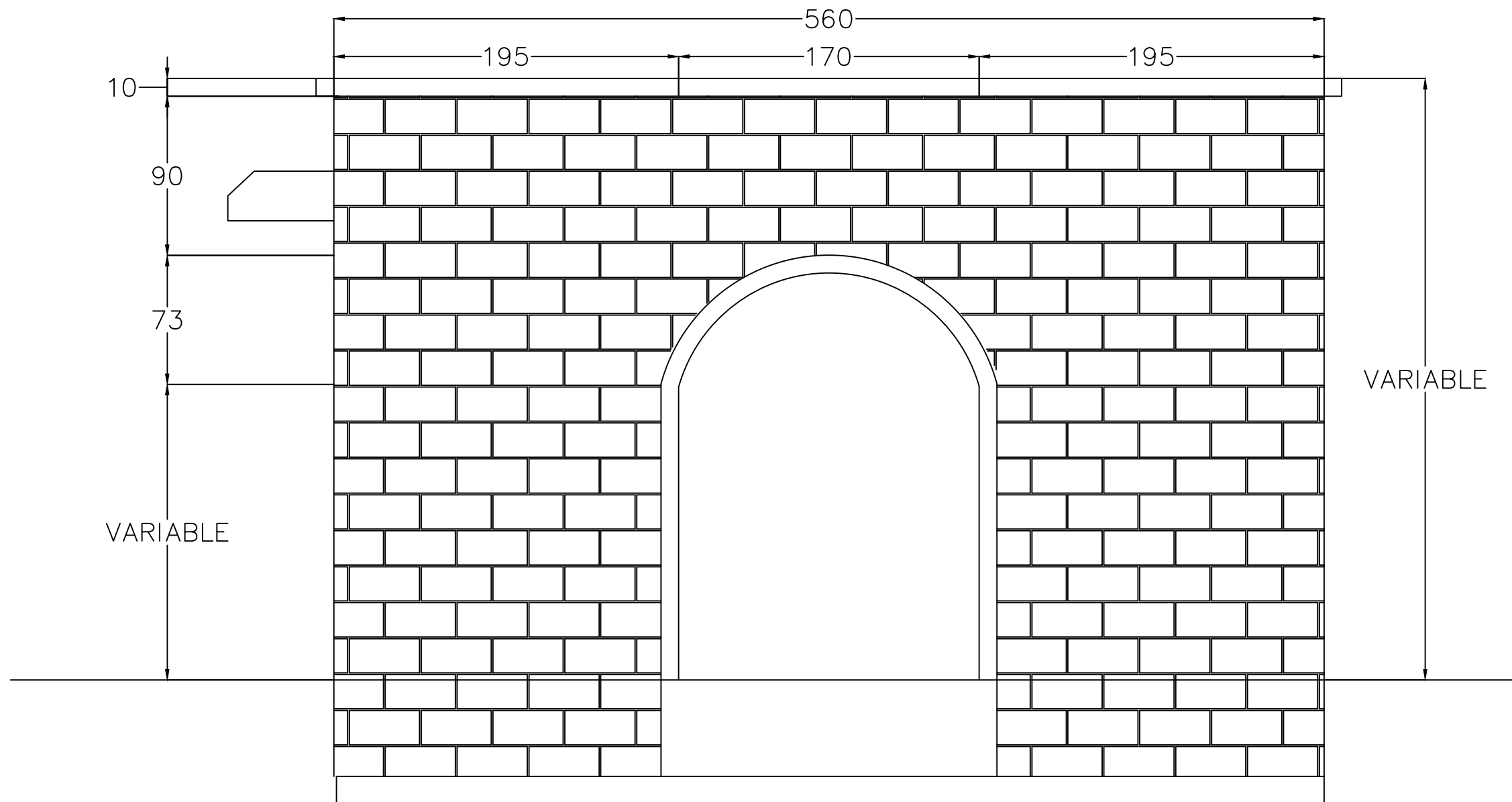
ESTRUCTURA DE PÓRTICO PR-01 ALZADO
