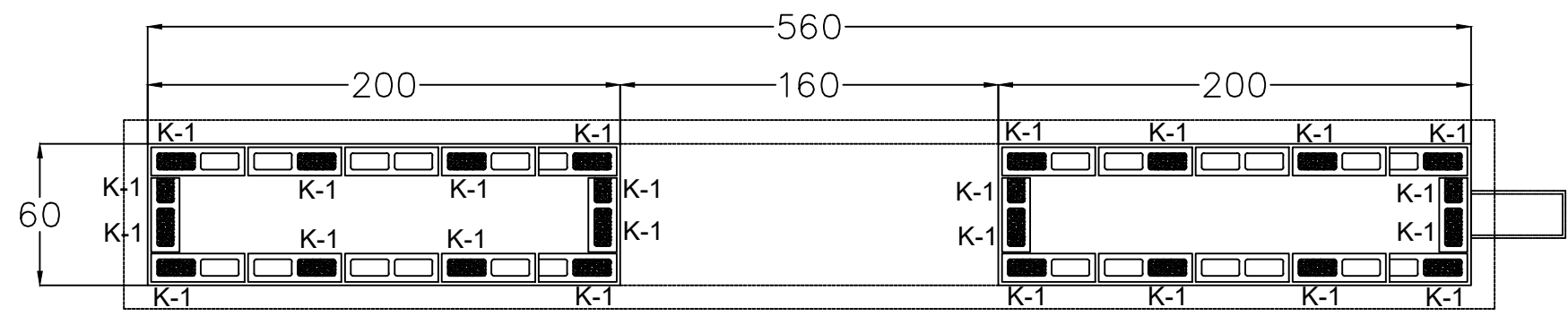
ESTRUCTURA DE PÓRTICO PR-01 PLANTA
