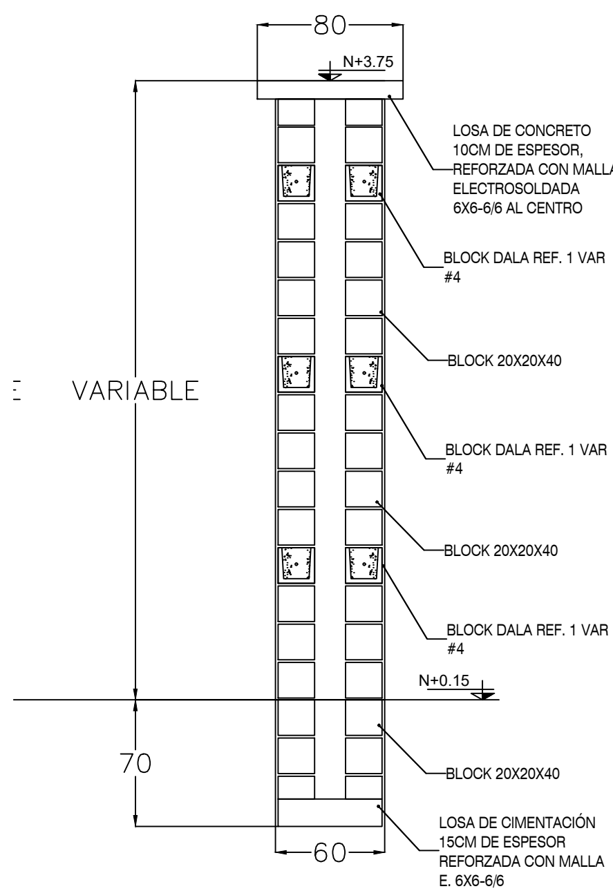
CORTE ESTRUCTURA DE PÓRTICO PR-01. ALZADO
